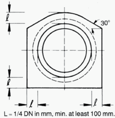
Fig. 12. Complete encasing
