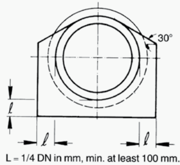
Fig. 11. Partial encasing
