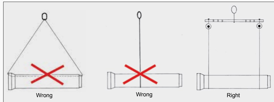
Fig. 3 Hoisting the pipe
